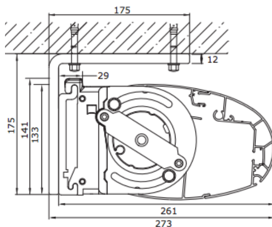
Plafondmontage
