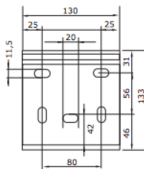
Vooraanzicht muursteun
